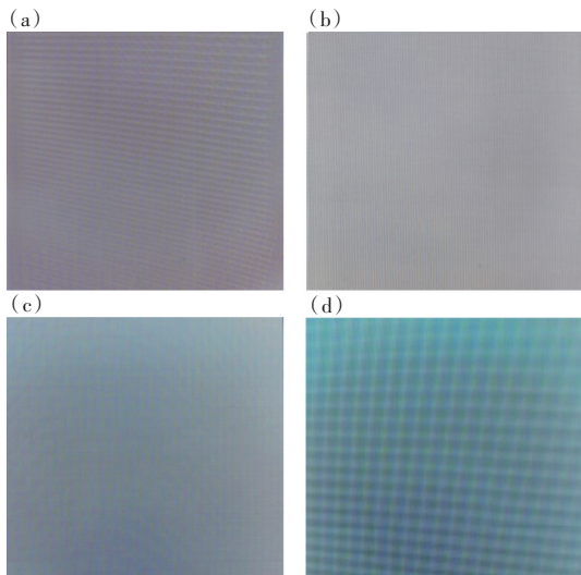
图10 (a)~(d)显示白场在-30,0,25,60℃时的LED实际显示效果。
